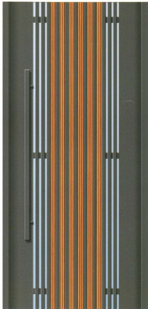
型號 F80 顏色 深灰砂紋 + 木紋鋁板 鉸鏈 旗型鉸鏈 門鎖 電鎖 材質 SECC
